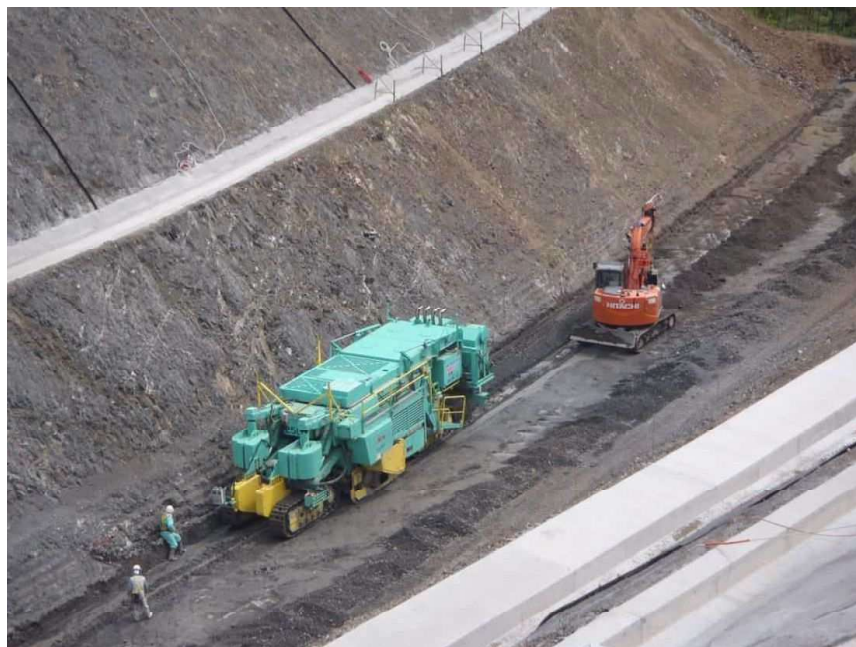
掘削状況
